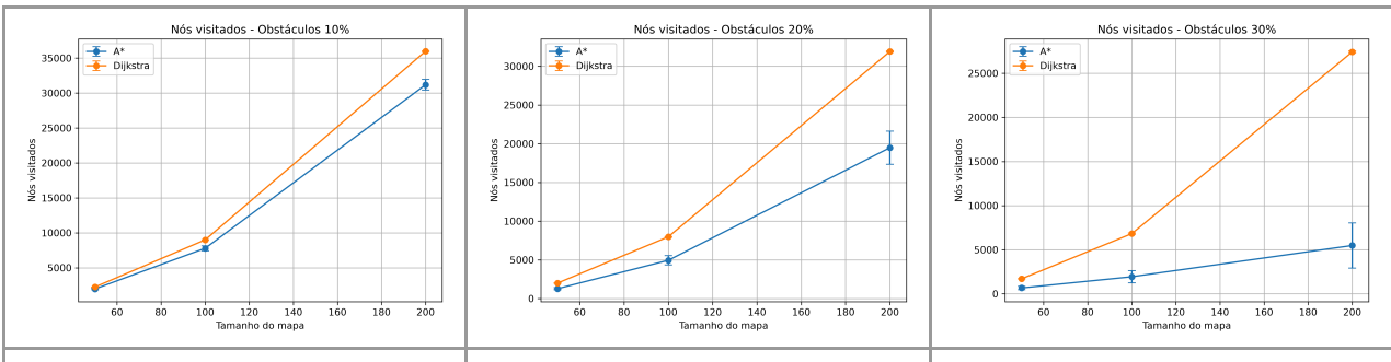
Figura 1. Nós visitados em função do tamanho do mapa para densidades de 10%, 20% e 30% de obstáculos (média ± desvio padrão sobre 30 sementes).
